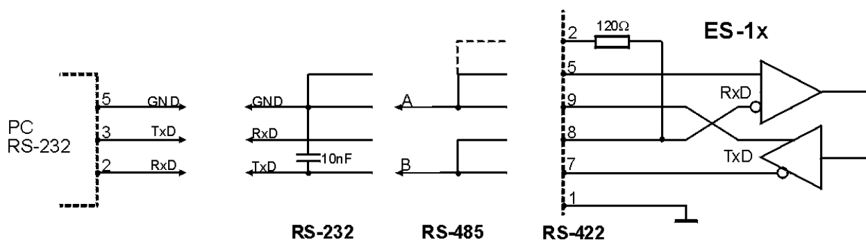
Rys. 1 Kanały szeregowo sterownika COM1 i COM2 (RS422/RS485/RS232)
