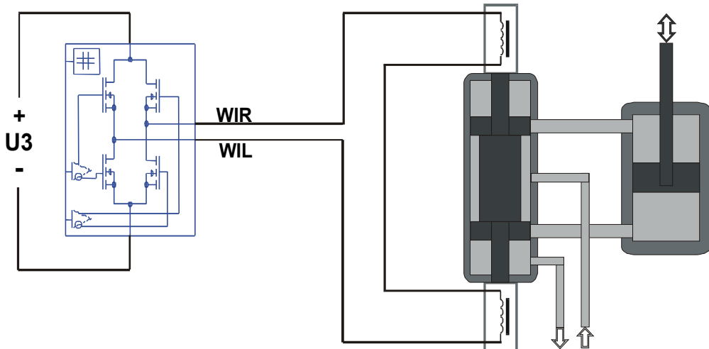
b) Obwód wykonawczy z cewkami połączonymi przeciwsośnie
